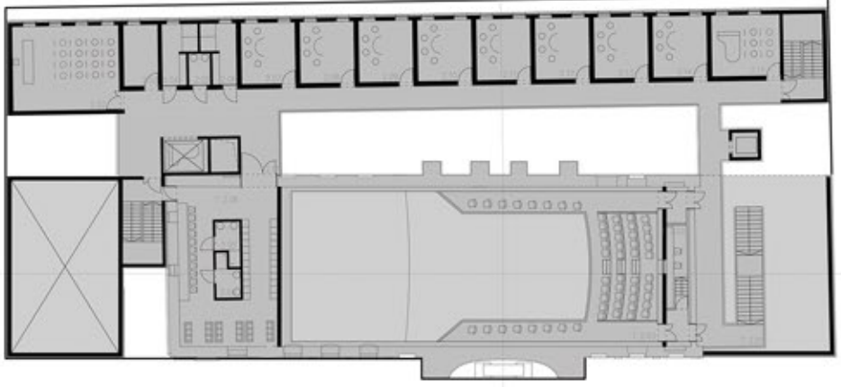
POZIOM 02 1:200
