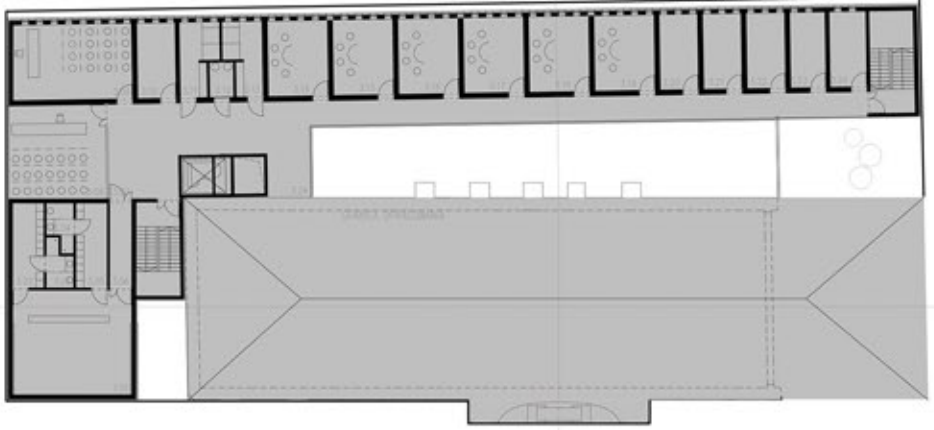
POZIOM 03 1:200
