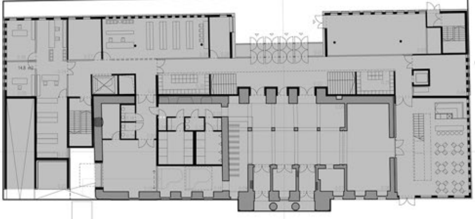
POZIOM 00 1:200
