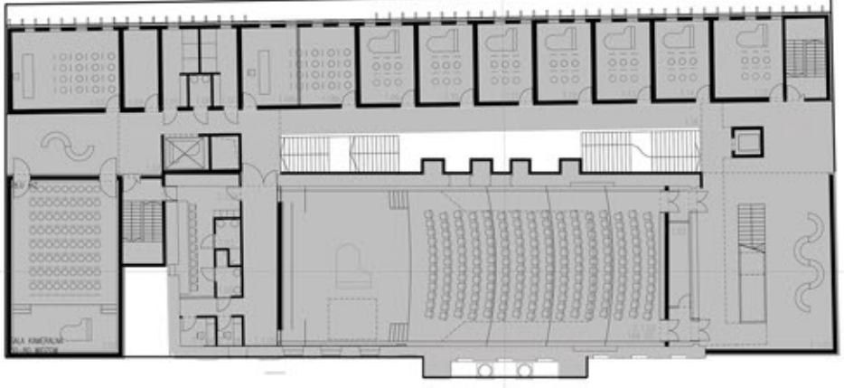
POZIOM 01 1:200
